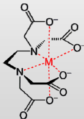
Metal-EDTA chelate
