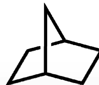
Norbornane
