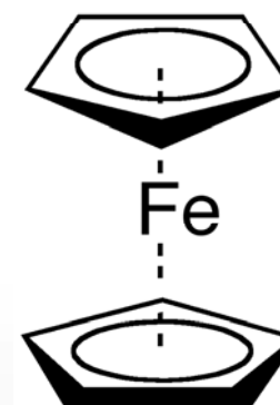
Ferrocene
